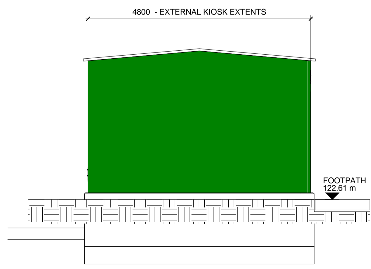
5 ELEVATION 'D' 1 : 50
