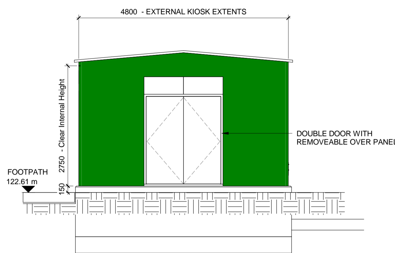
4 ELEVATION 'C' 1 : 50
