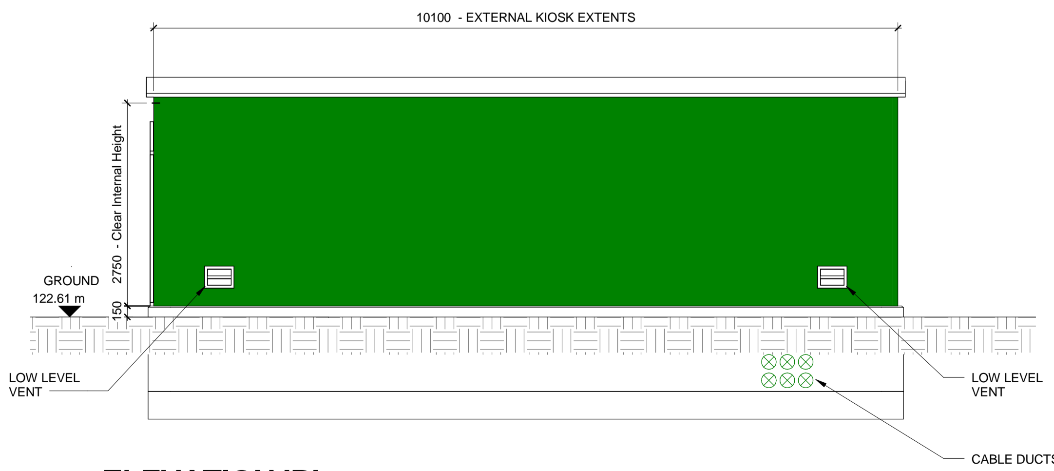
3 ELEVATION 'B' 1 : 50
