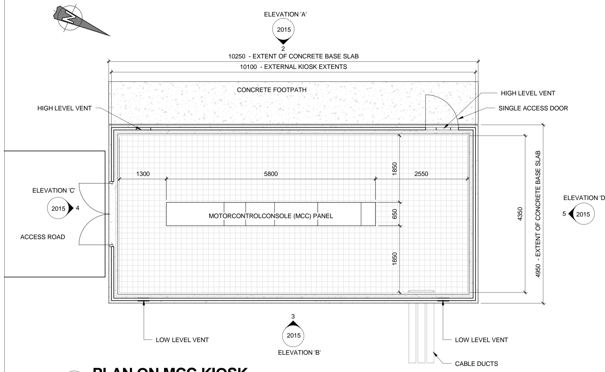
1 PLAN ON MCC KIOSK 1 : 50
