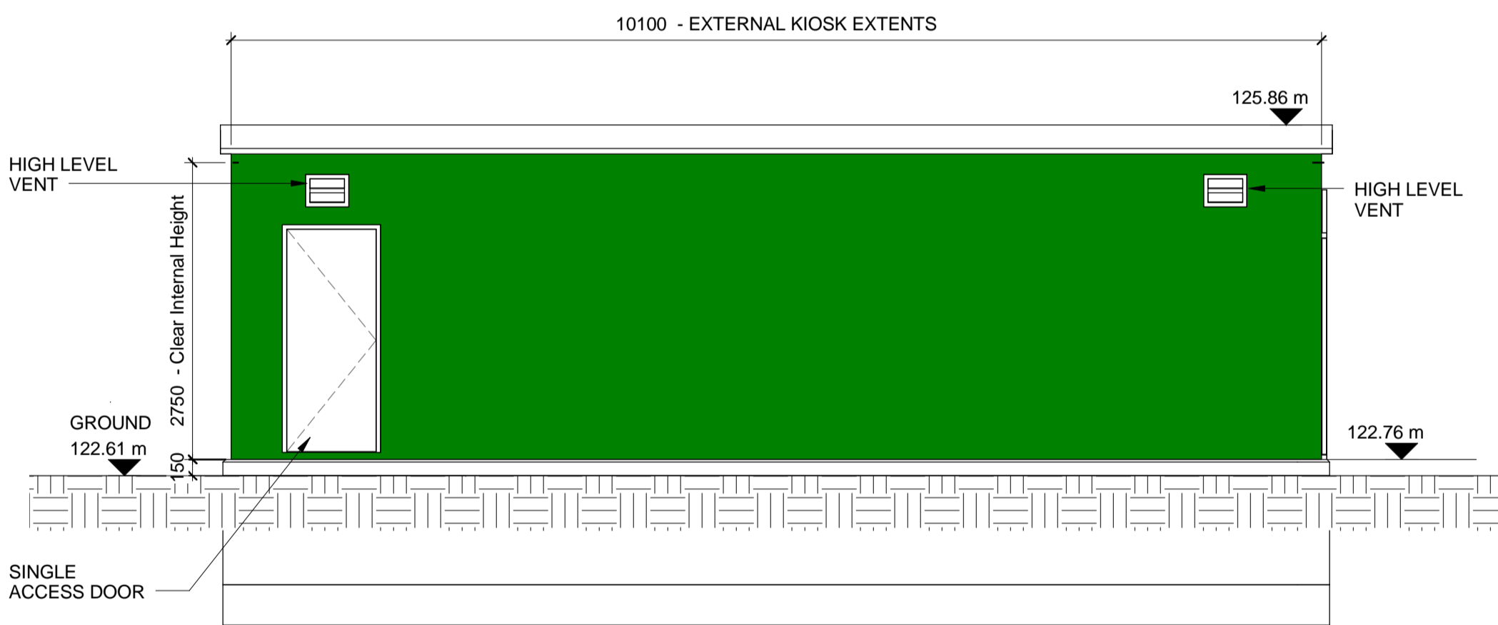
2 ELEVATION 'A' 1 : 50
