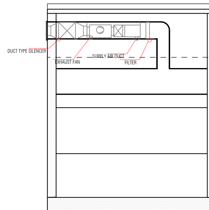
A-A SECTION /scale 1:50/
