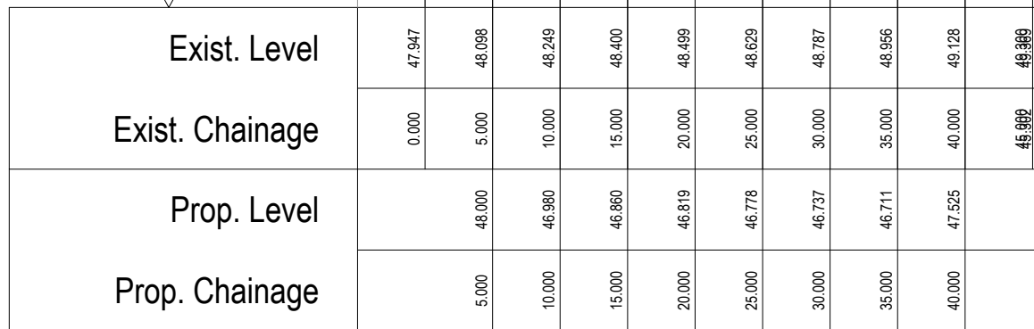
BASIN A-A Horiz. 1:500 Vert. 1:100 45.00 A.O.D.
