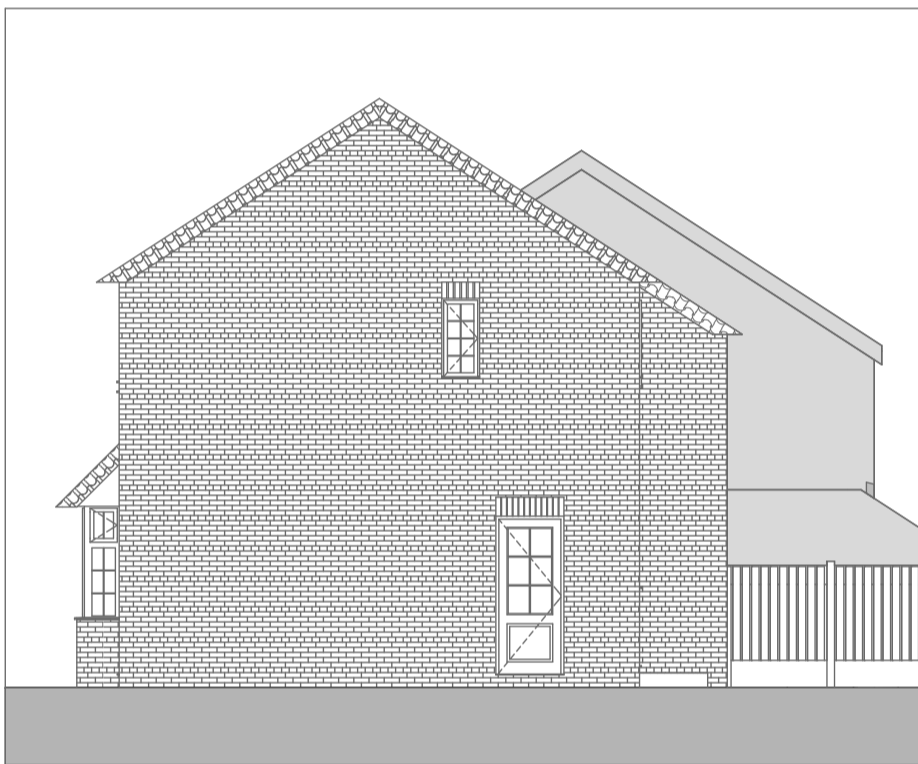
E-02 Elevation 1:100
