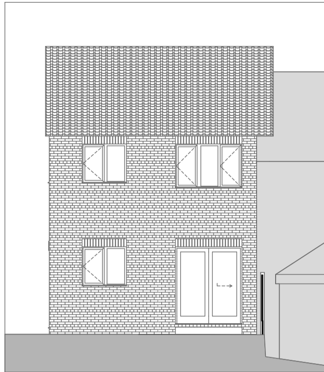
E-03 Elevation 1:100
