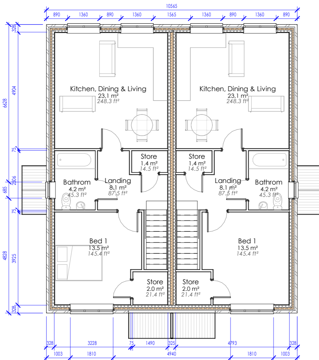
2 | *L01 - AP A/B 1 : 100
