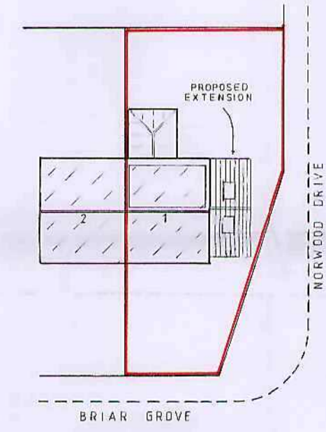
SITE PLAN 1:250
