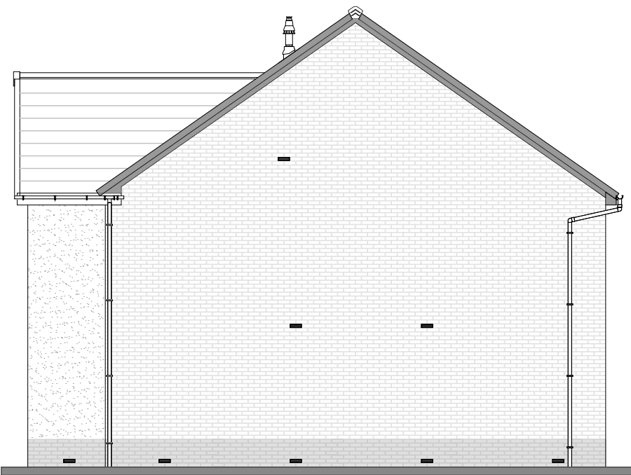
RIGHT ELEVATION
