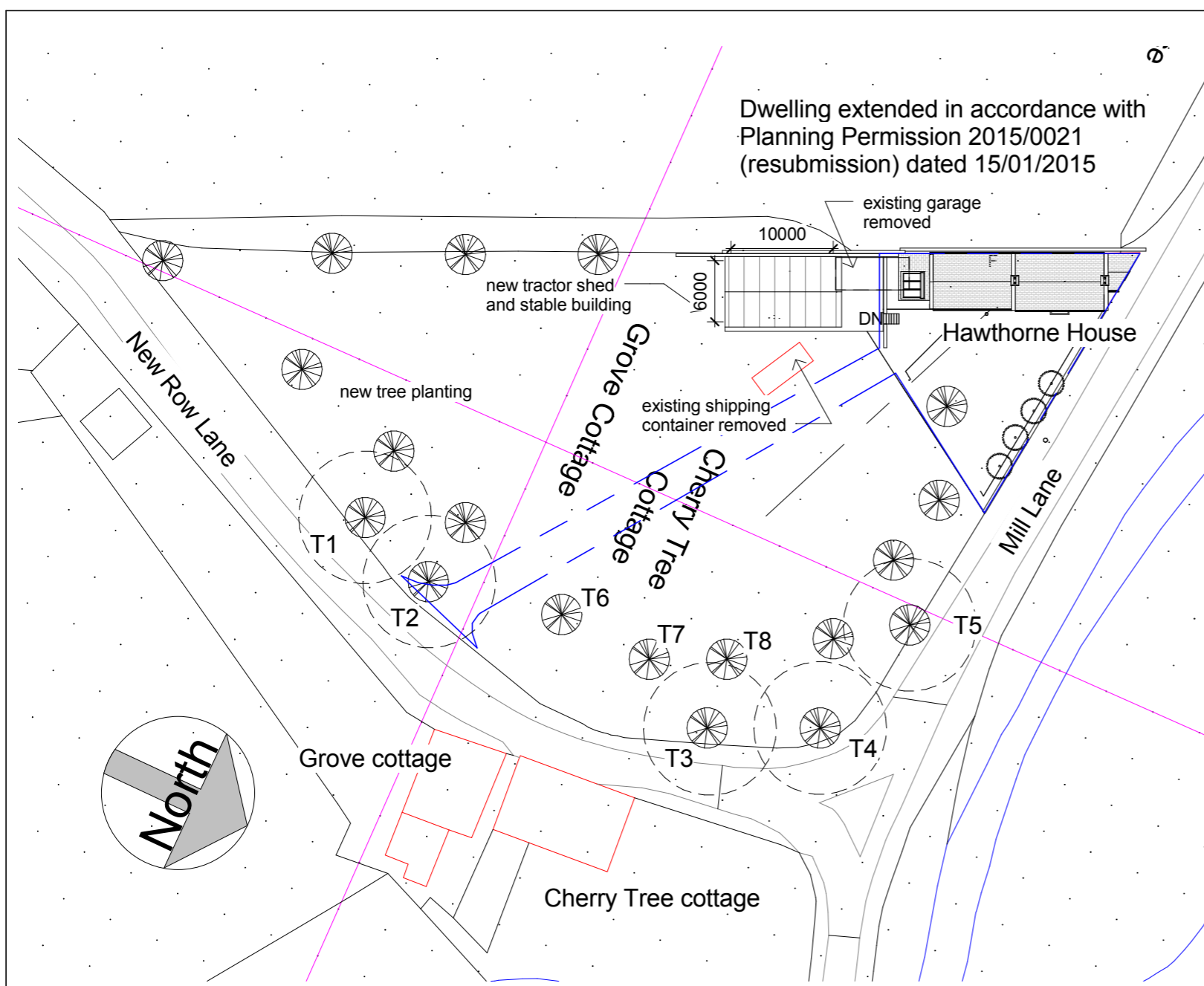
2 Site 1 : 500
