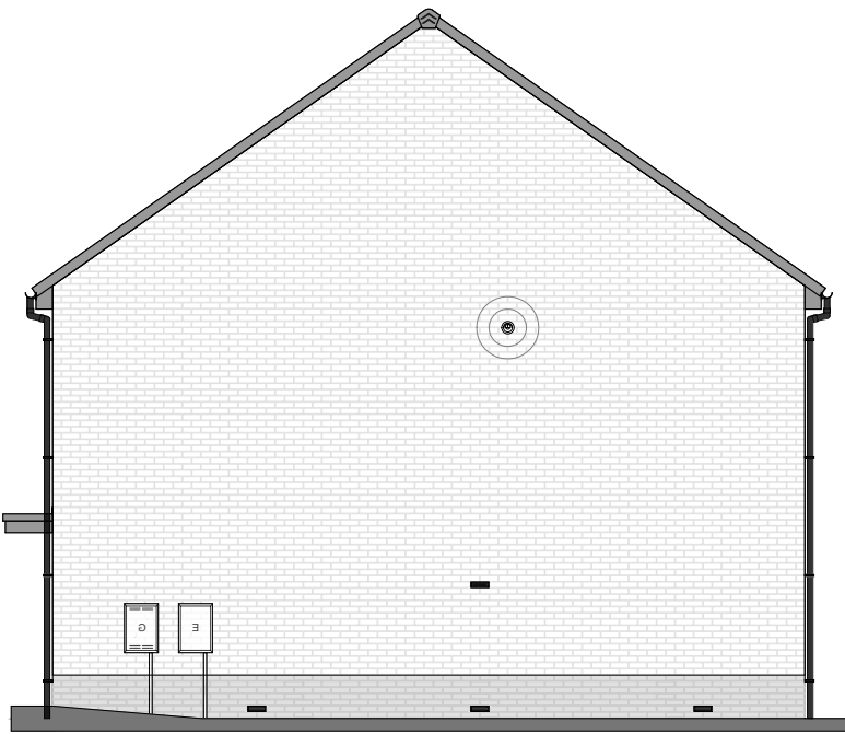
RIGHT ELEVATION
