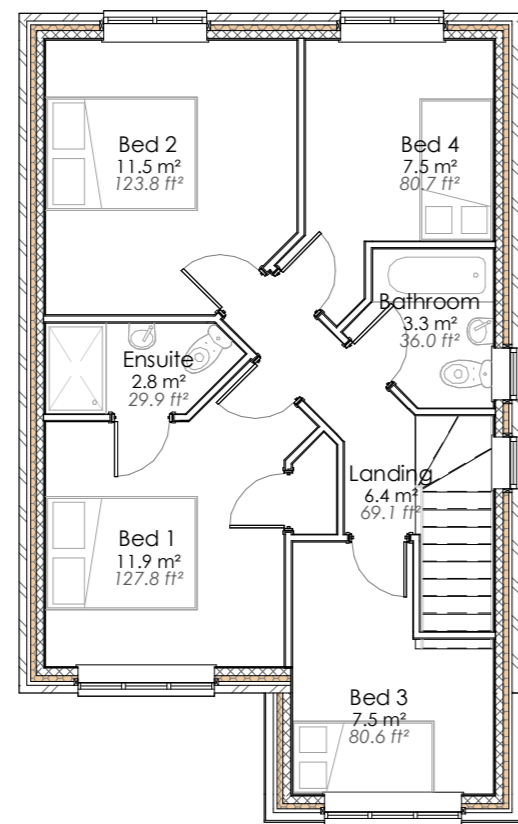
2 | *L01 - HTE 1 : 100
