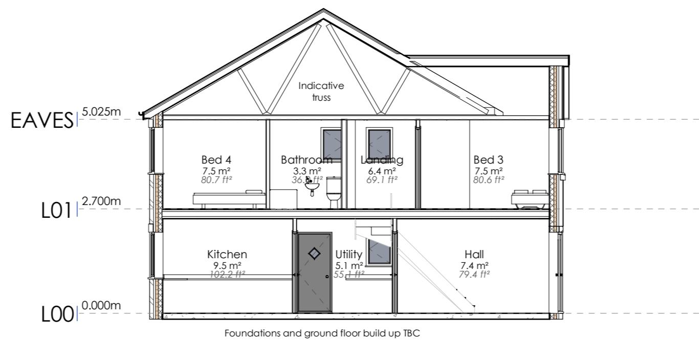
7 | HTE Section 1 : 100
