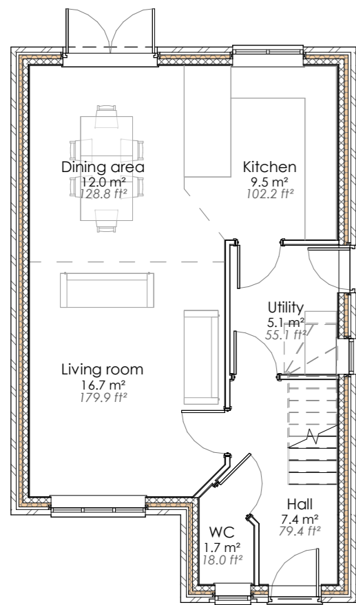
1 | *L00 - HTE 1 : 100
