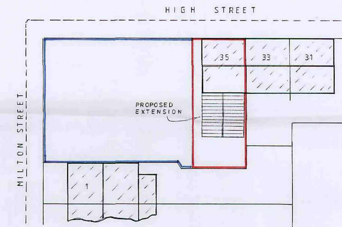
SITE PLAN 1:250
