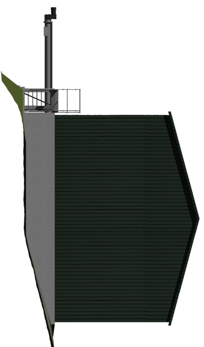
Elevation B 1:1:00
