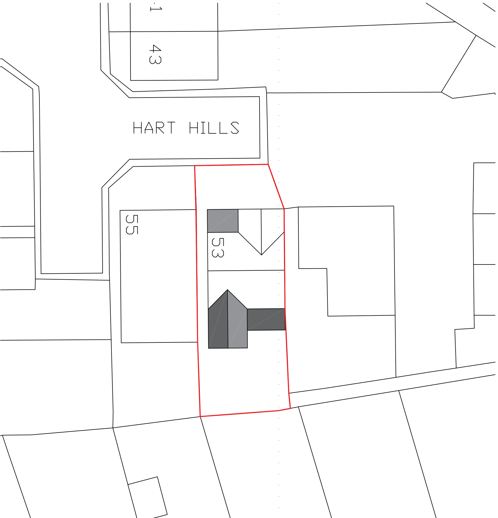
Site Plan 1:200
