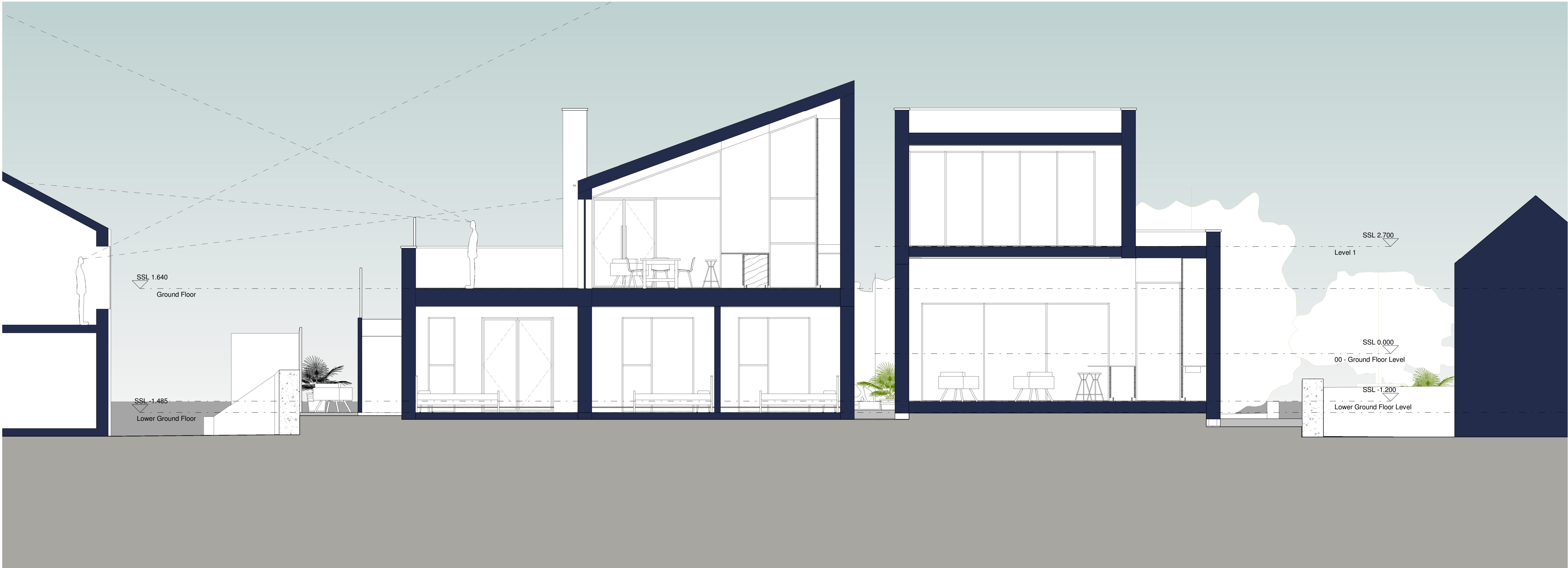
Site Section 1 : 50
