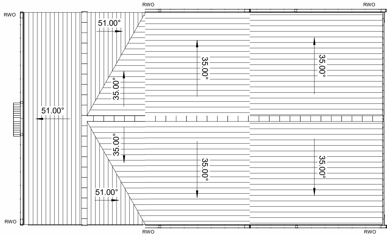
Roof Plan 1 : 100
