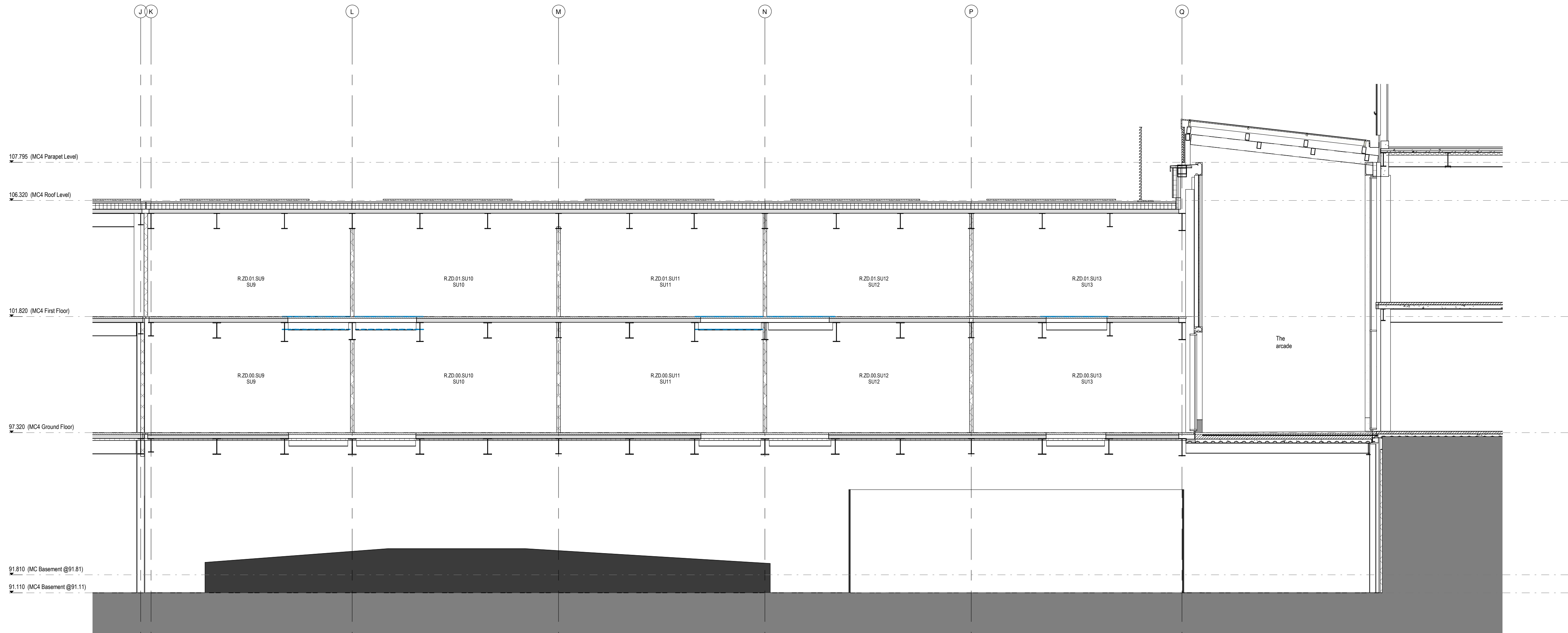
B1 Section BB GL A-J 1 : 100
