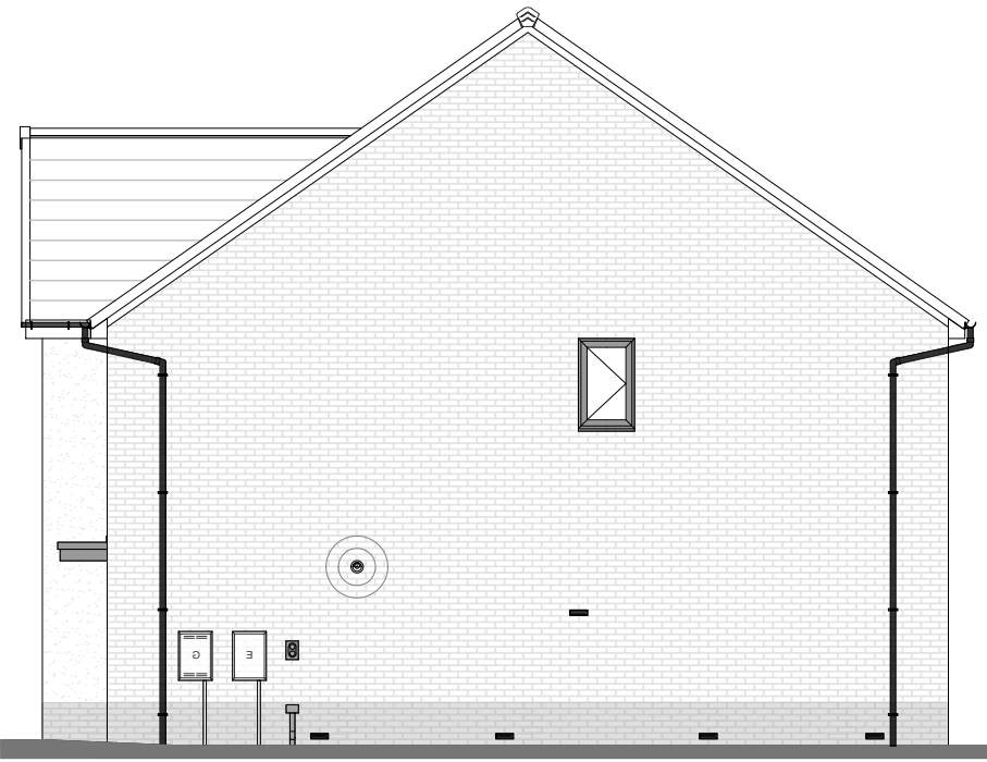
RIGHT ELEVATION
