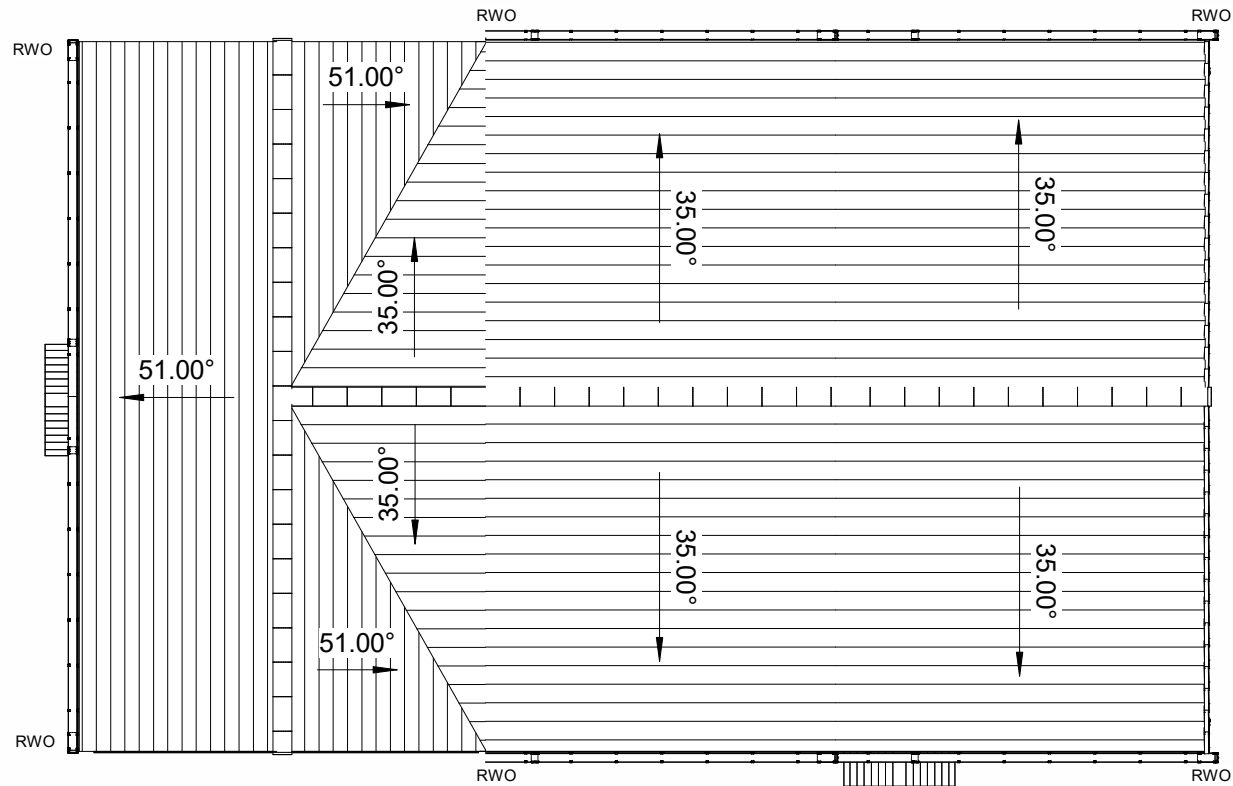
Roof Plan 1 : 100
