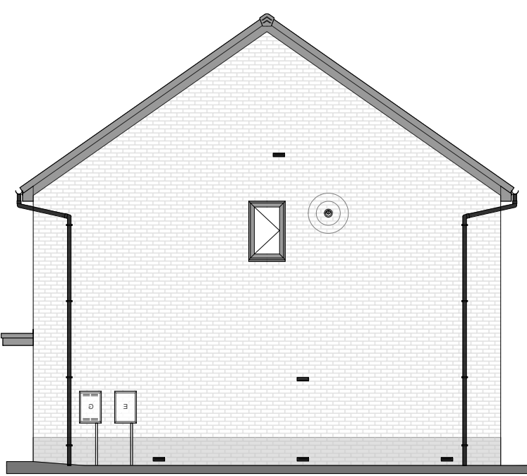
RIGHT ELEVATION
