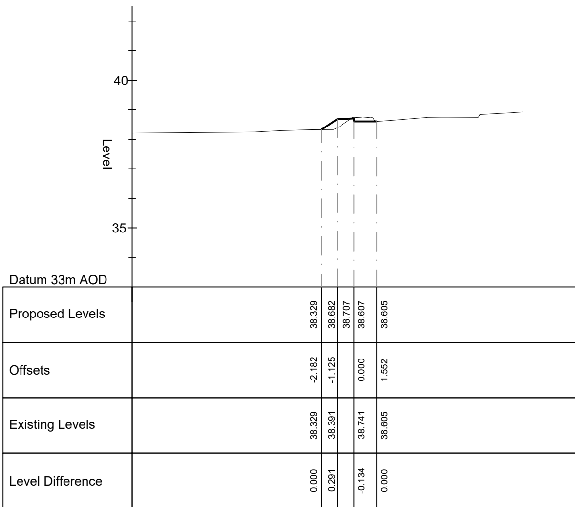
Chainage 20.000
