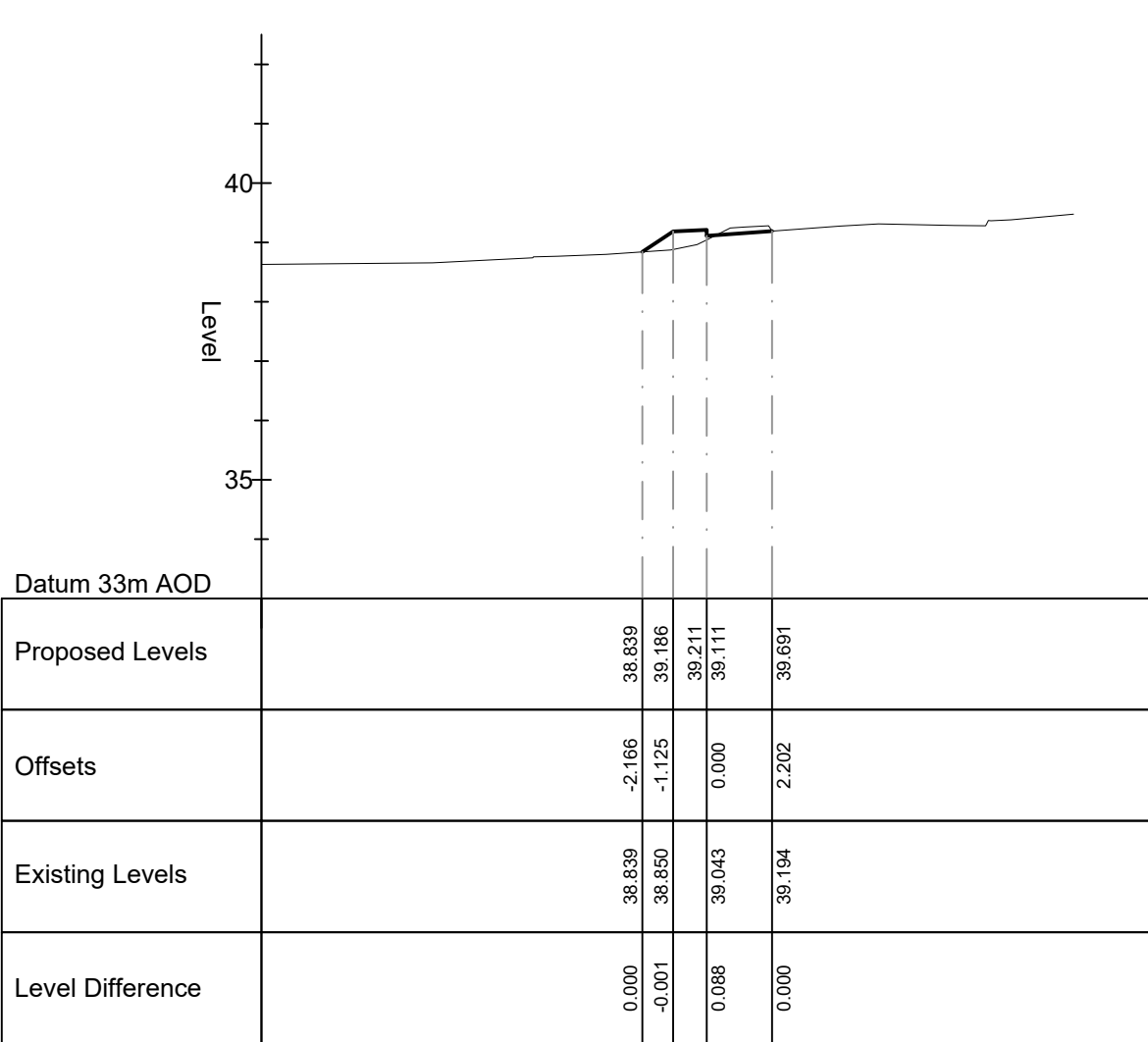
Chainage 30.000
