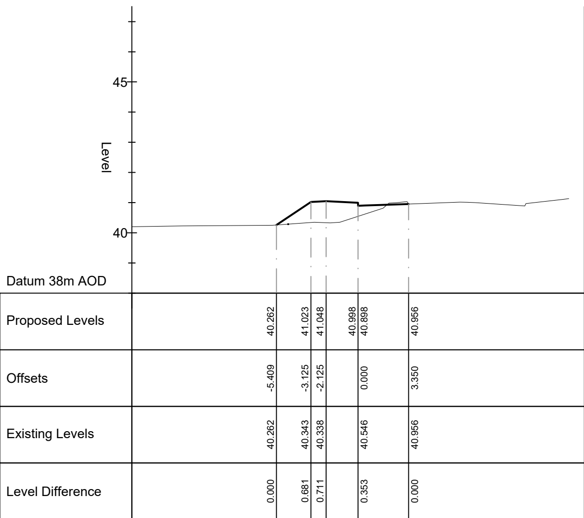
Chainage 60.000
