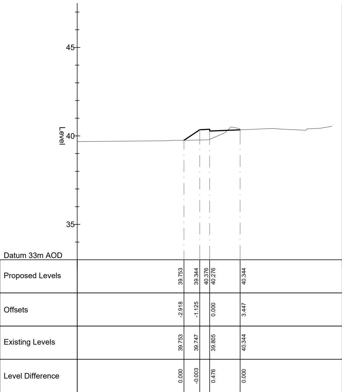
Chainage 50.000
