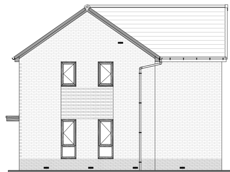
RIGHT ELEVATION
