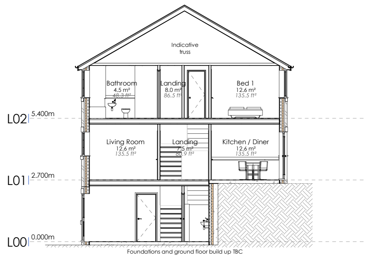
8 | HTA3 Section 1 : 100
