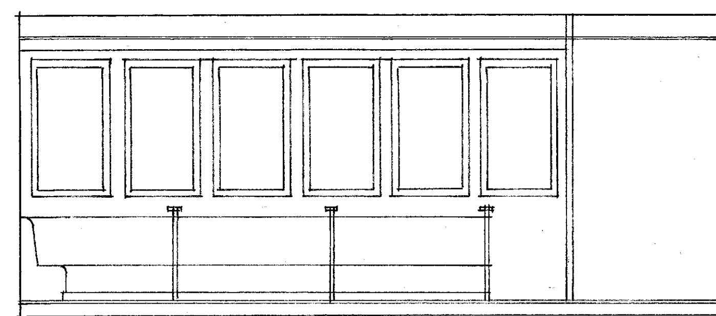
ELEVATION A
