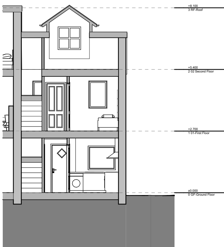
4 Section DD 1:100
