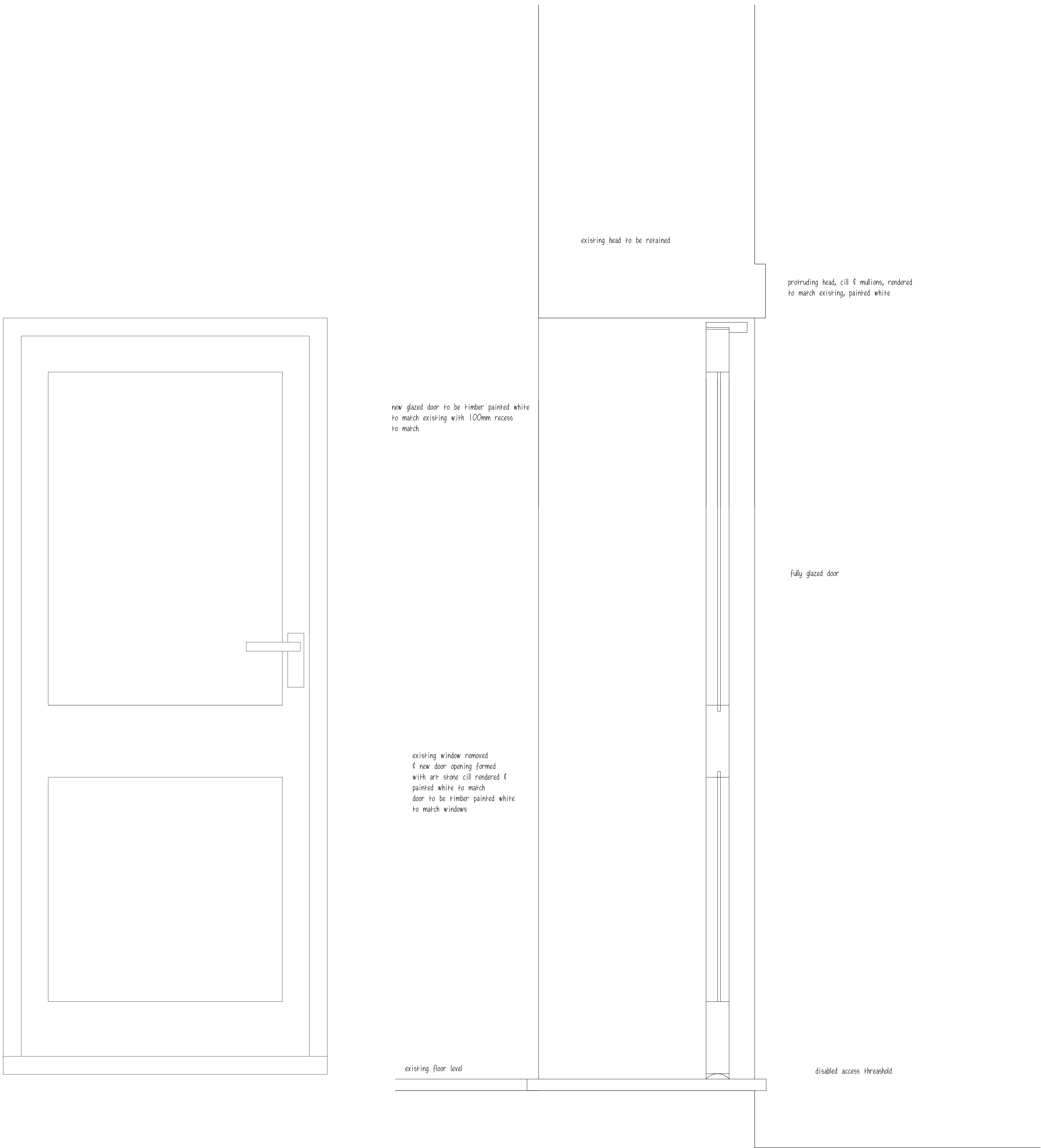
SECTION THRO DOOR
