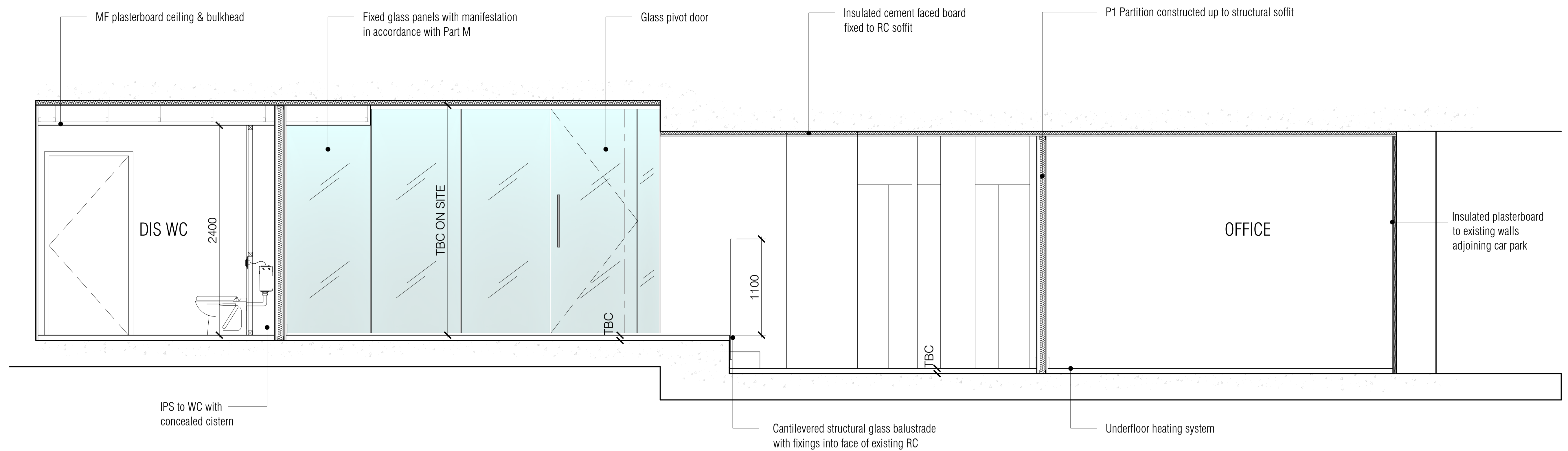
SECTION A-A
