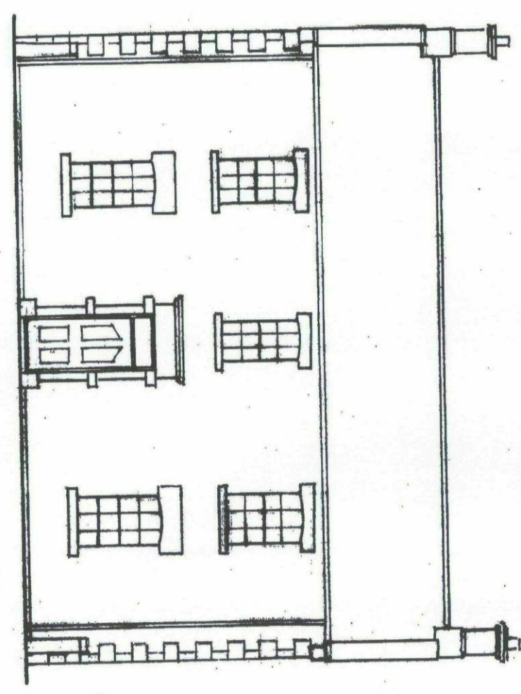
FRONT ELEVATION N.W.
