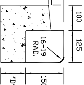
SECTION D-D
