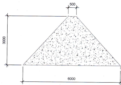
1 Bund Section 1 : 50
