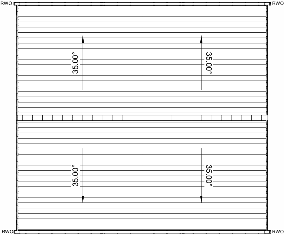
Roof Plan 1 : 100
