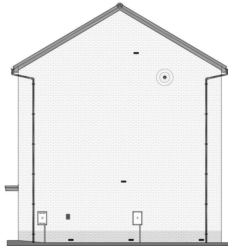
RIGHT ELEVATION
