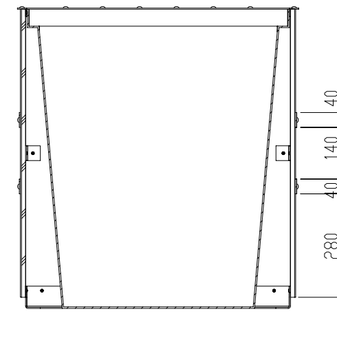
COUPE A-A
