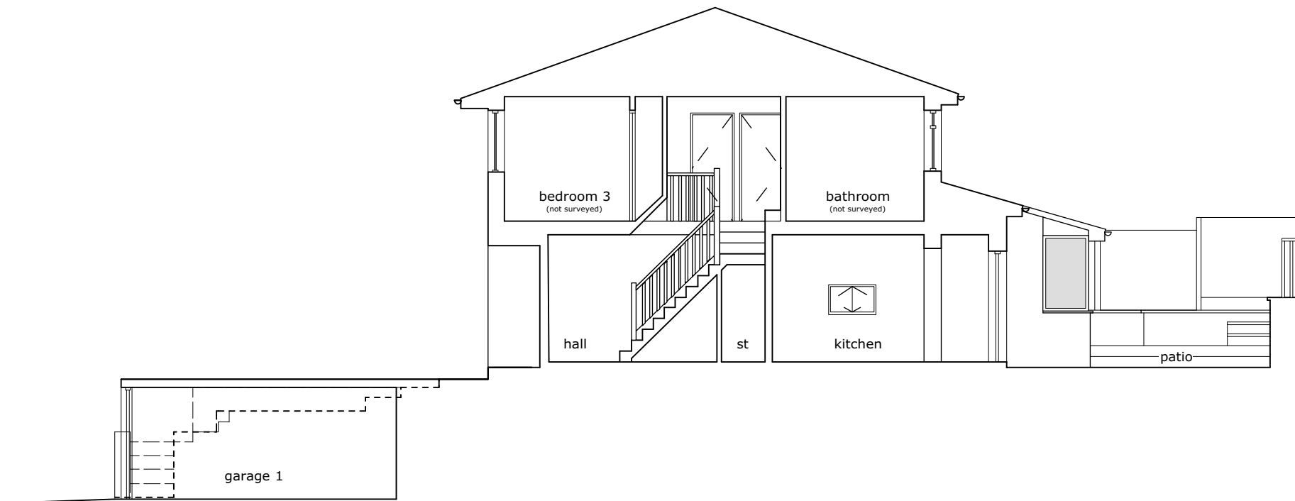
section A-A
