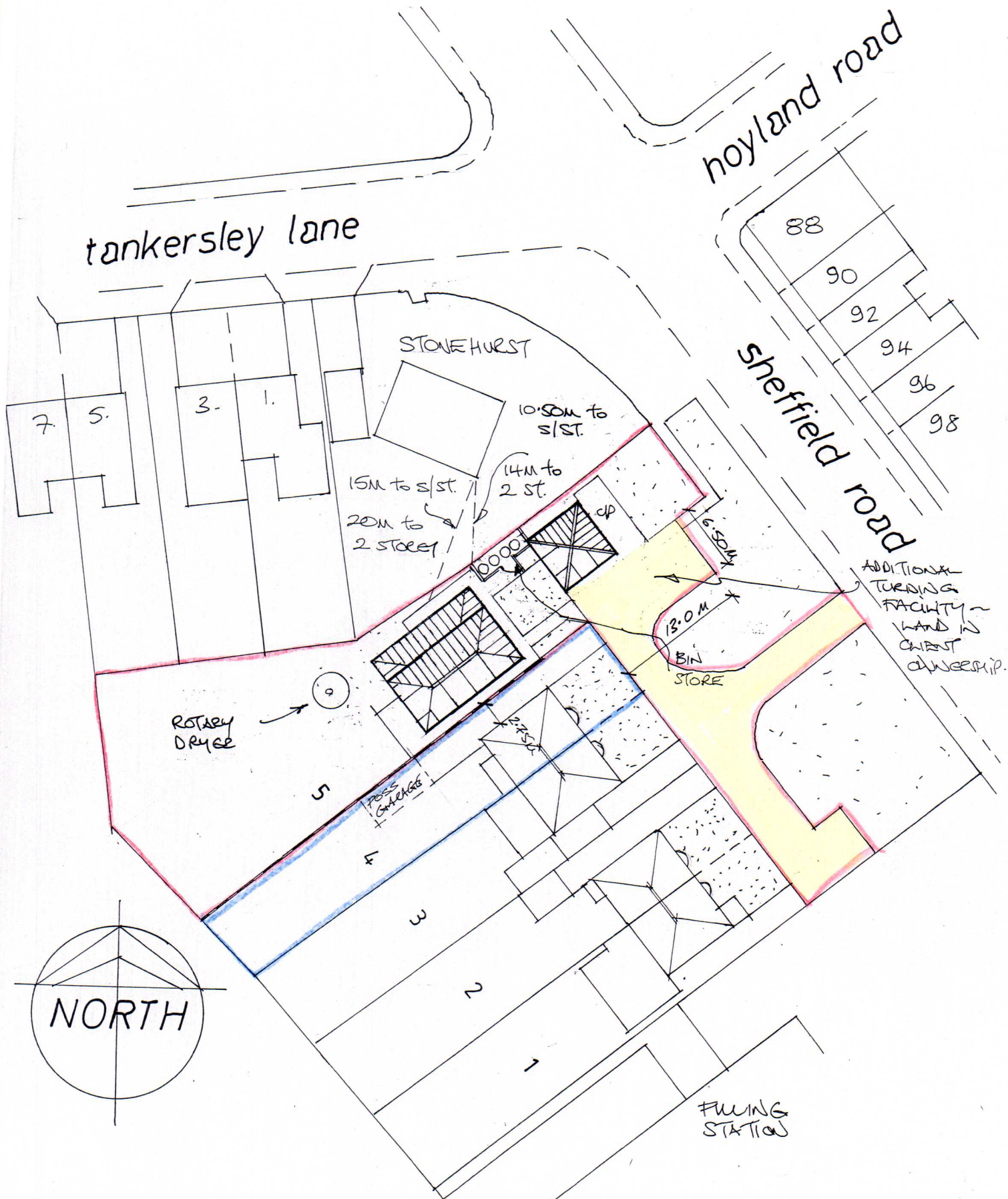
Site Layout 1:500
