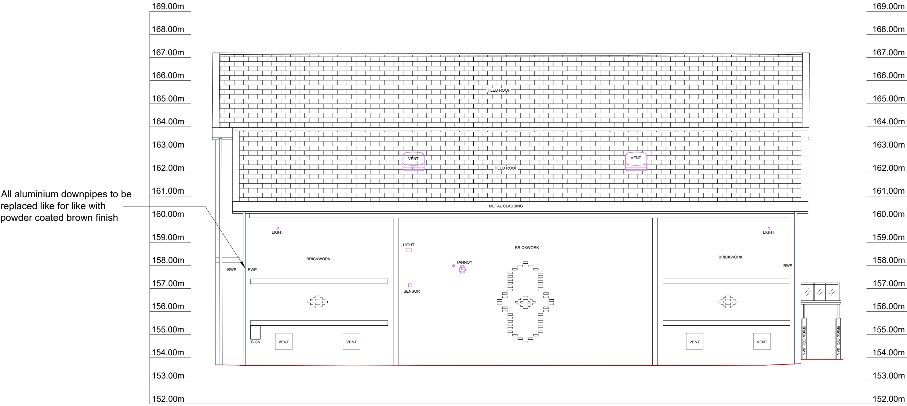
ELEVATION 4 1:100
