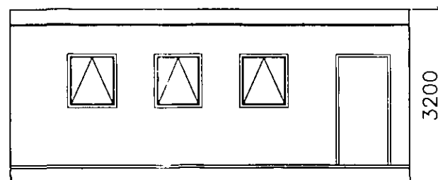
Elevation B
