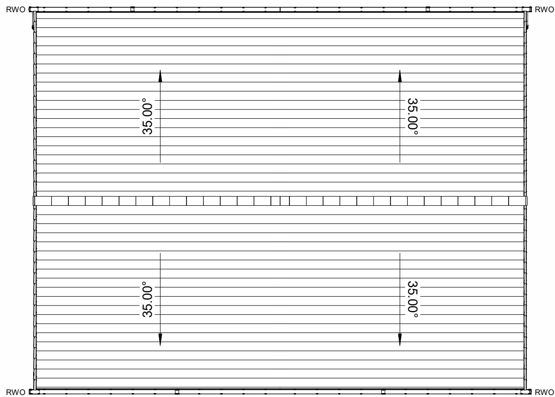
Roof Plan 1 : 100
