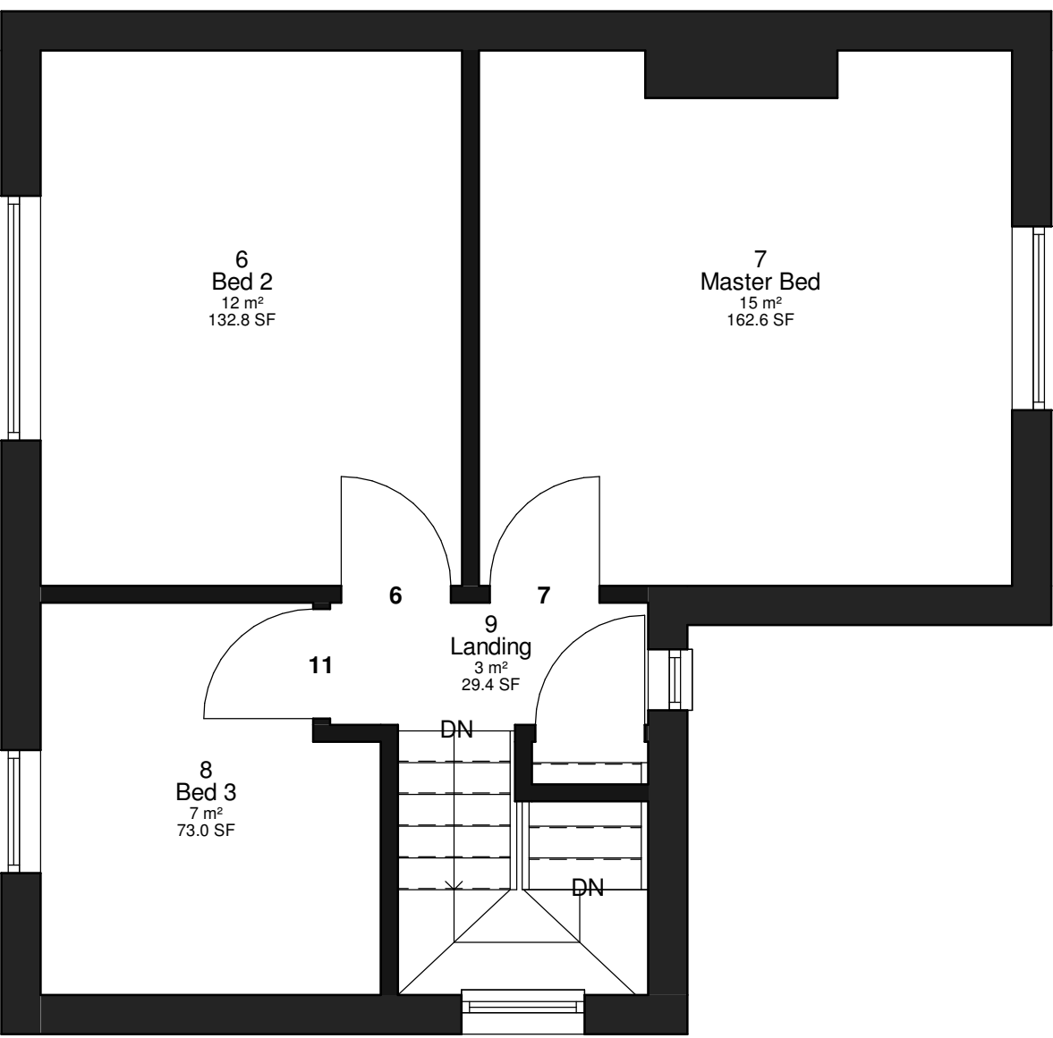
Level 1 1 : 50
