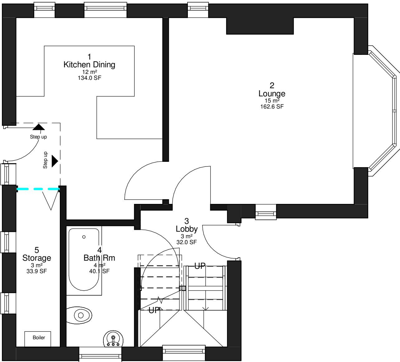
Level 0 1 : 50
