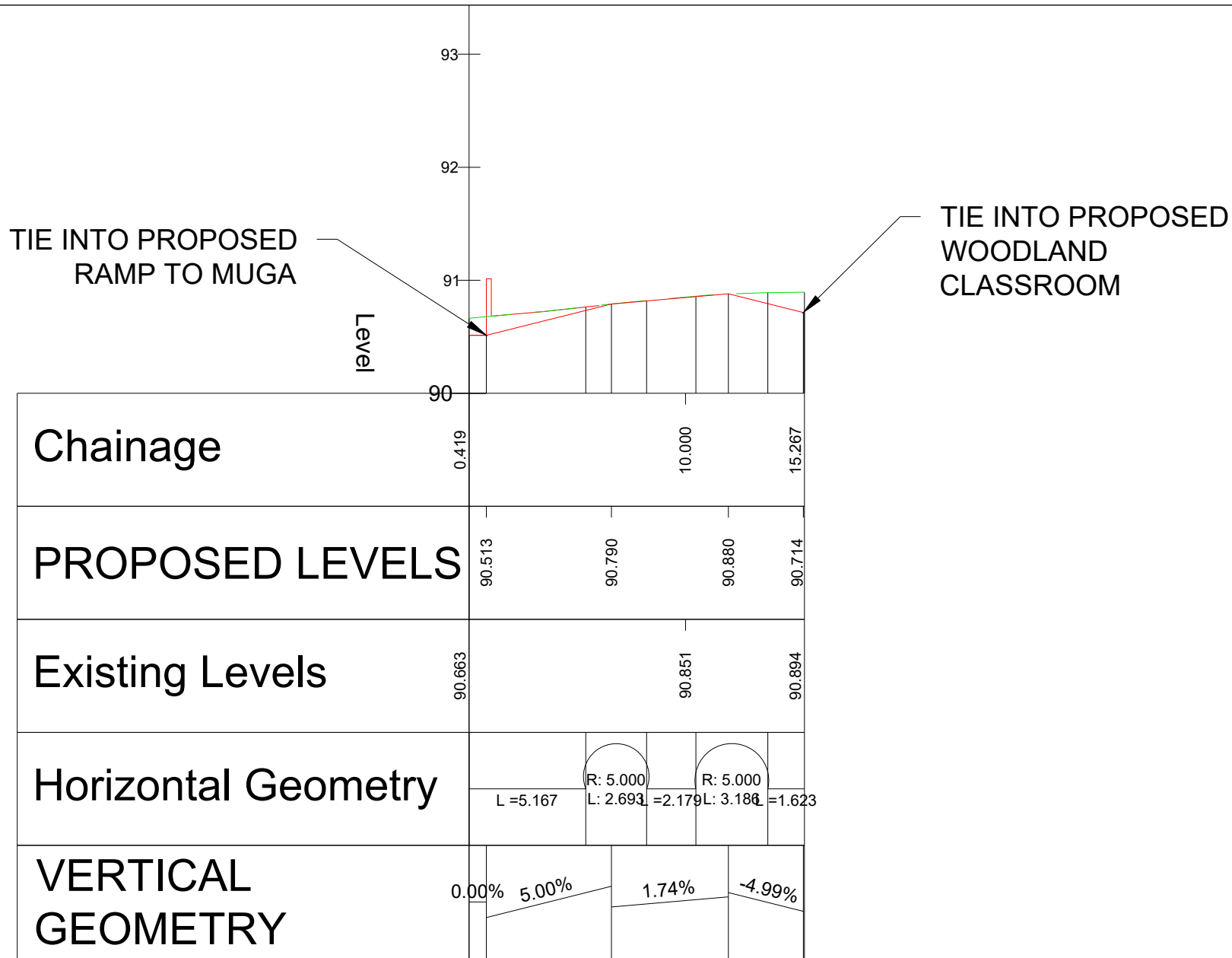
WOODLAND LINK - LONG SECTION SCALE: H 1:200,V 1:40. DATUM: 90.000
