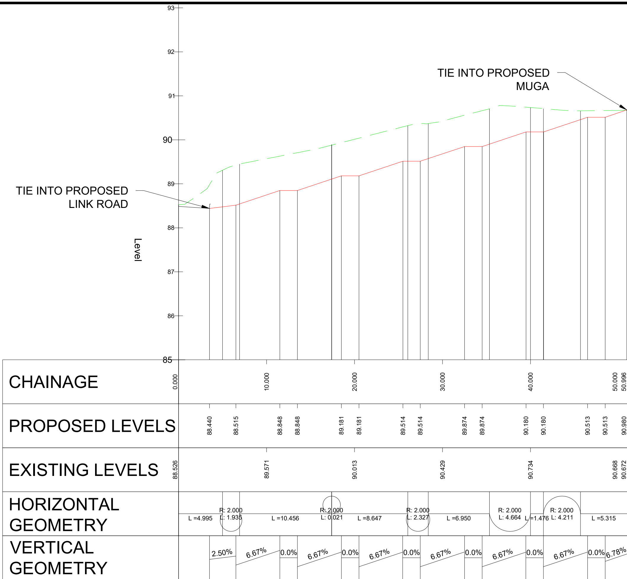
ALIGNMENT - DDA RAMP 2 - LONG SECTION SCALE: H 1:200,V 1:40. DATUM: 85.000
