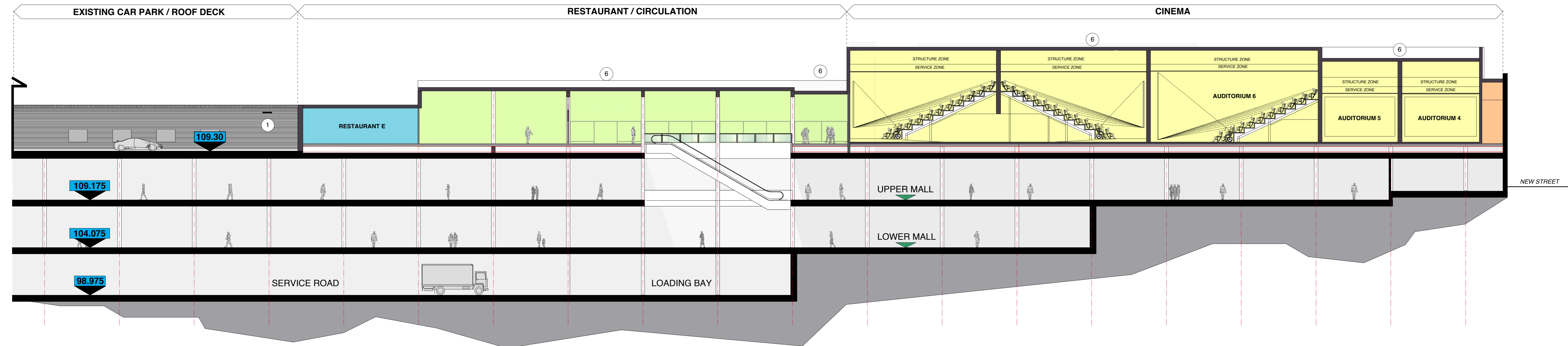
SECTION A-A
