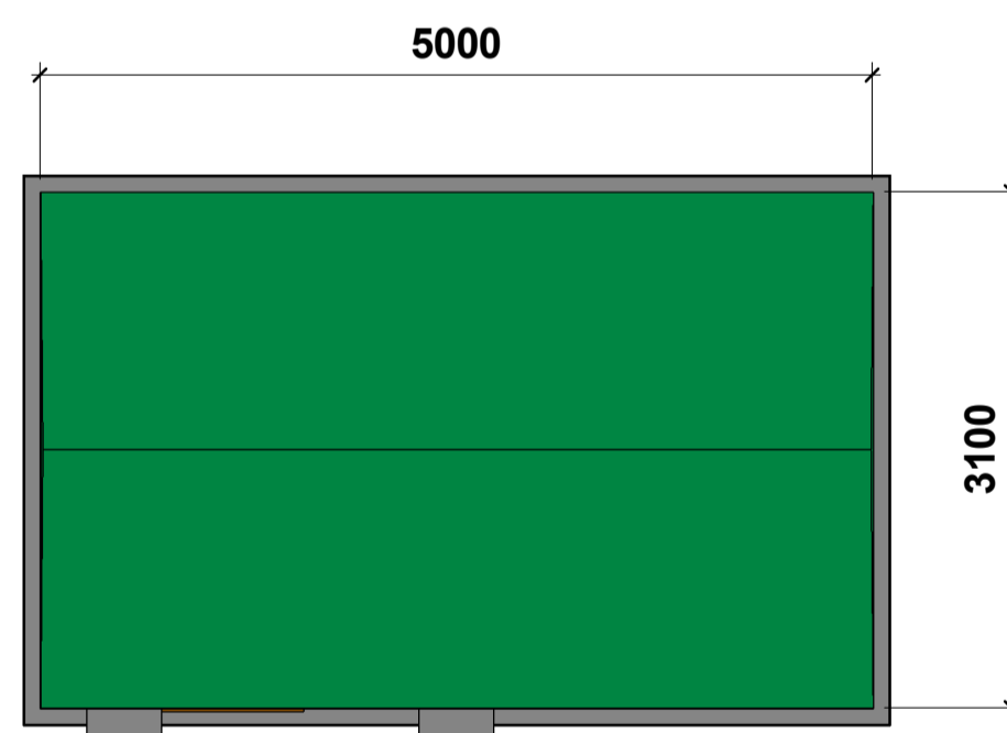
Plan 1 : 50
