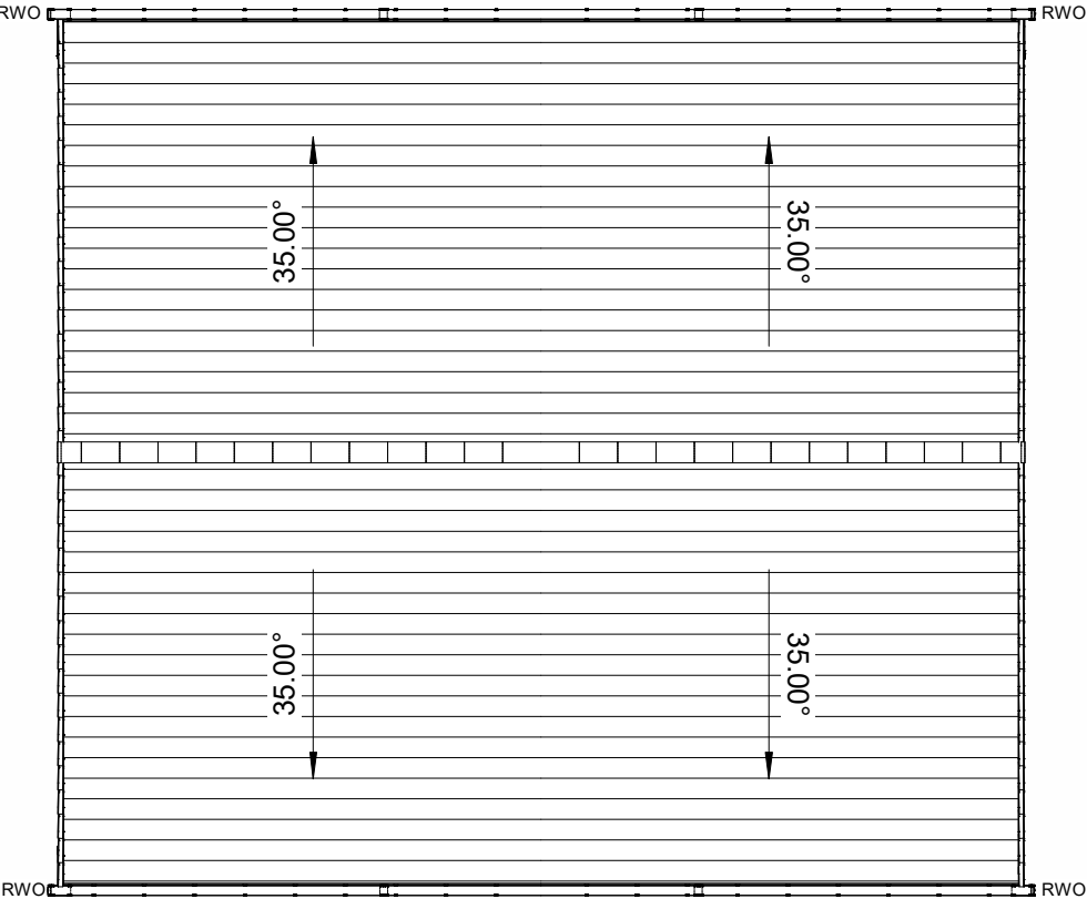
Roof Plan 1 : 100
