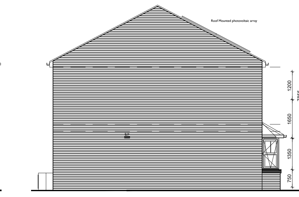
End Elevation
