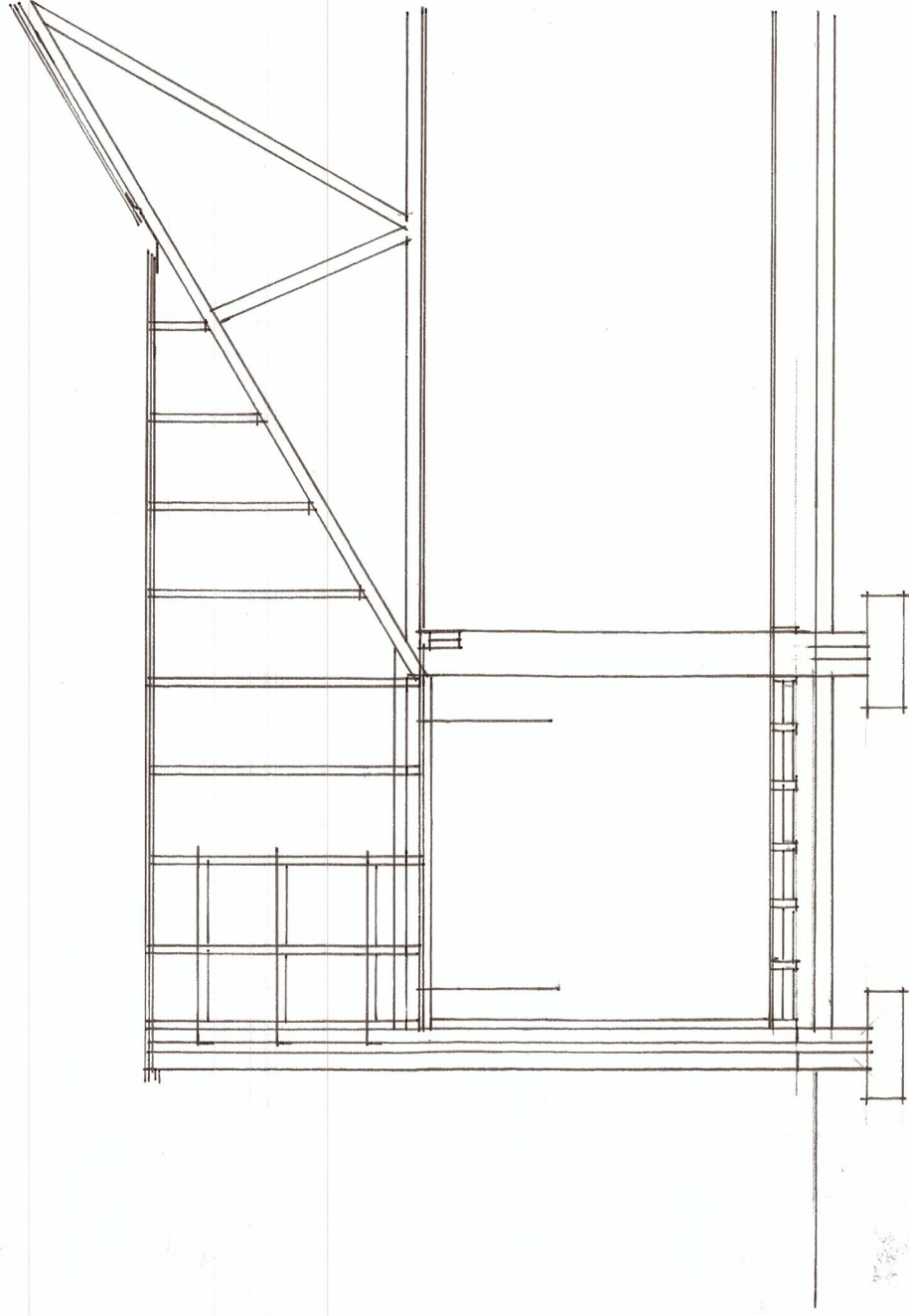
SECTION BB 1:50
