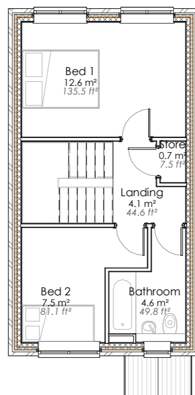
2 | *L01 - HTA 1 : 100
