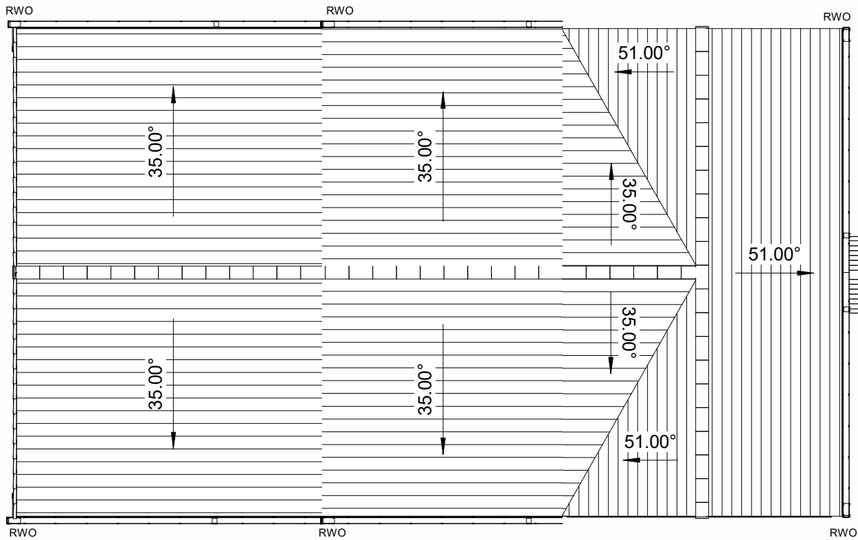
Roof Plan 1 : 100
