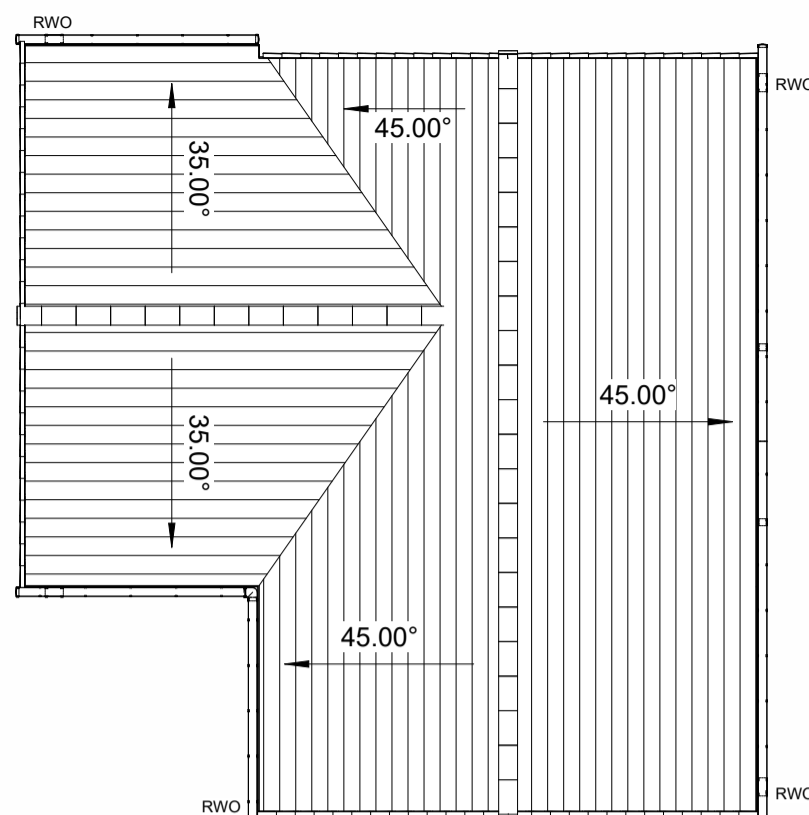
Roof Plan 1 : 100
