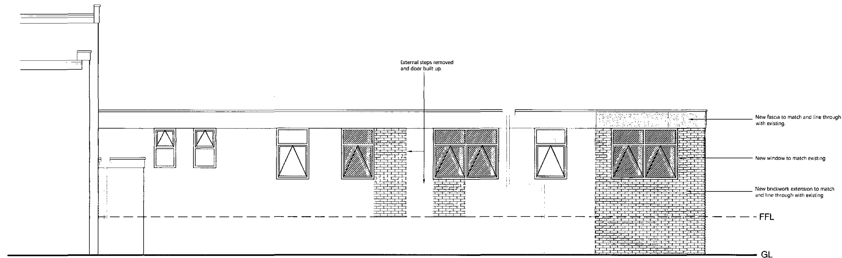
ELEVATION B
